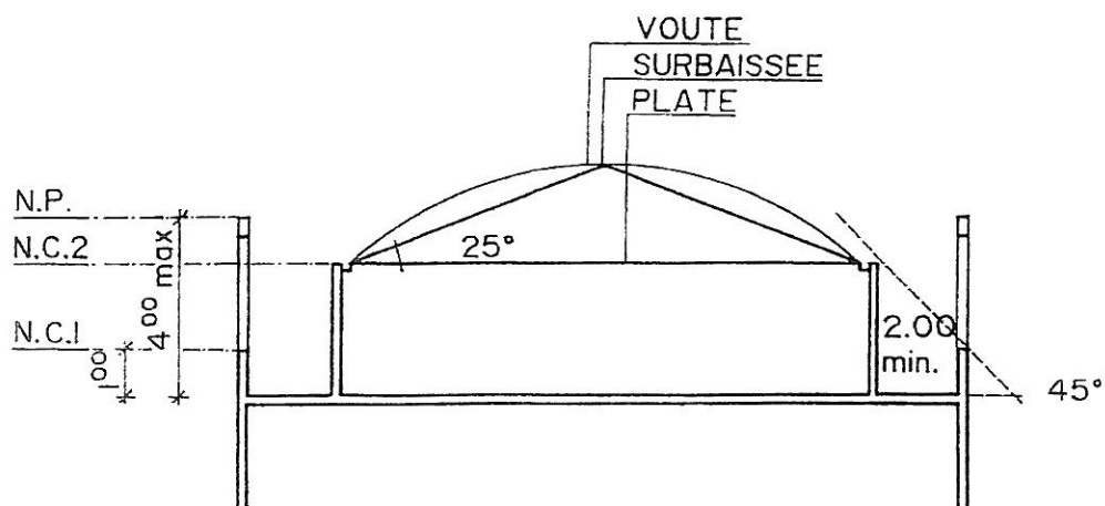
COUPE ETAGE EN RETRAIT
